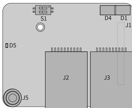
图1-3 MD500-PN1卡接口布局
