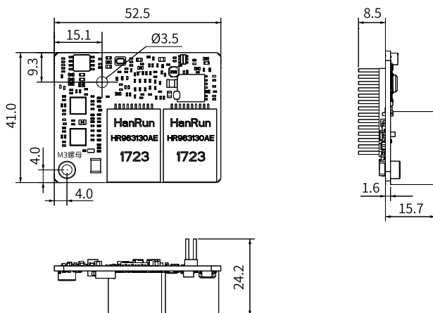
图1-2 MD500-PN1卡尺寸图（单位：mm）
