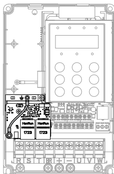
图2-2 MD500-PN1卡和变频器接地连接示意图
