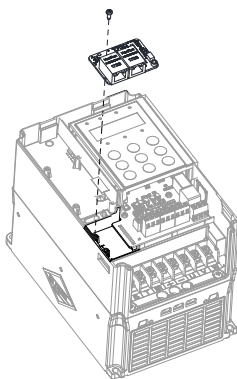
图2-1 MD500-PN1卡安装示意图
